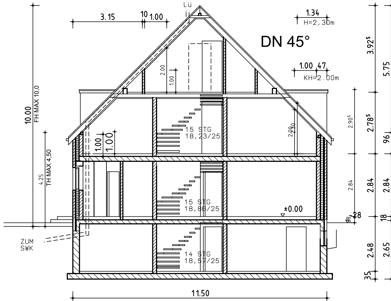
SCHNITT WOHNHAUS
