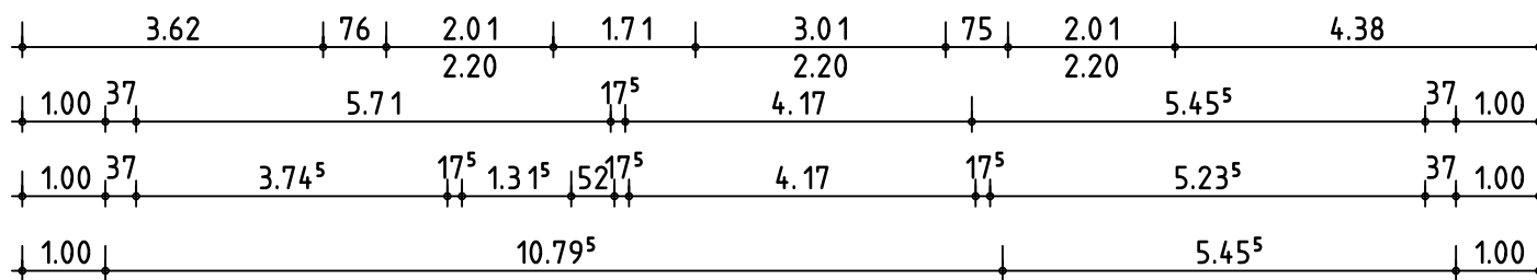
GRUNDRISS 2. OBERGESCHOSS
